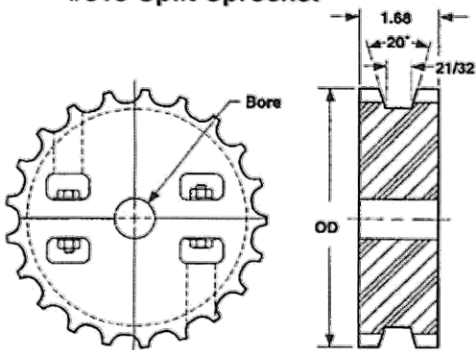
820 Sprocket - Split
