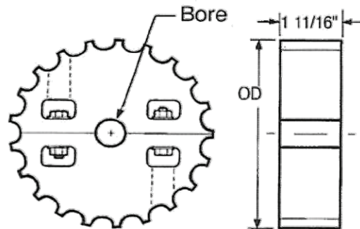
#815 Split Sprocket
