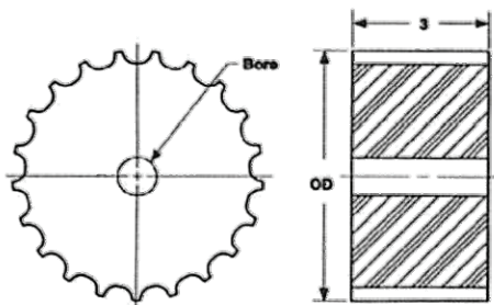
821 Sprocket
